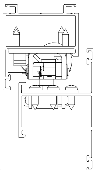
Ouvrant extérieur
