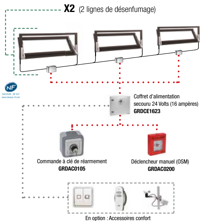
Standard électrique (vérins)
